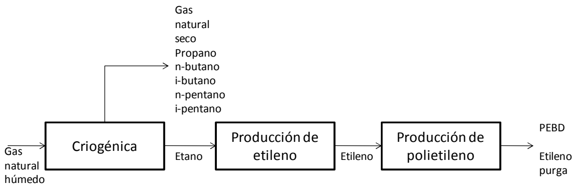
Figura A2.1. Cadena de producción de polietileno de baja densidad a partir de GNH (el eteno se conoce coloquialmente como etileno)
