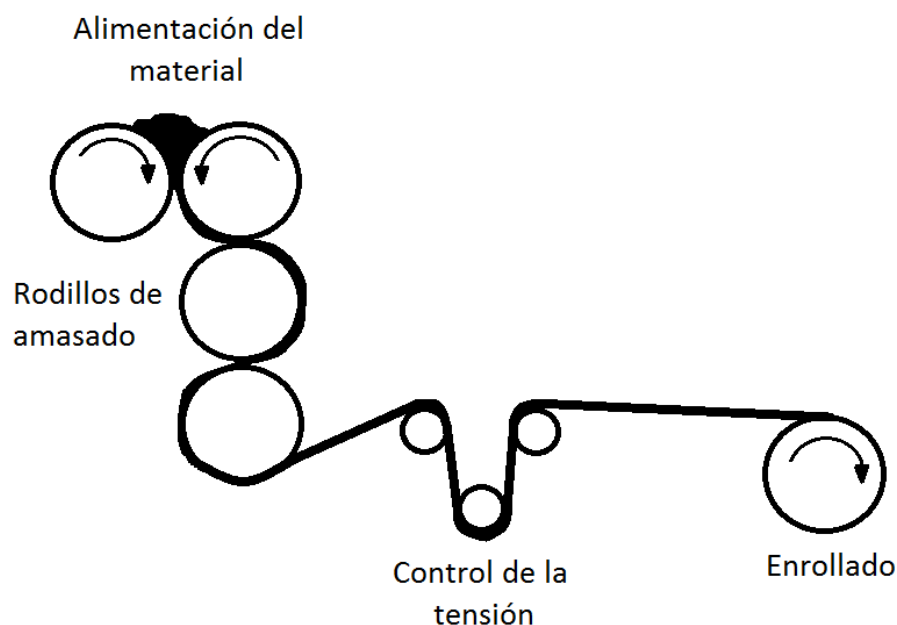
Figura A1.4. Proceso de “calandreo”. Fuente: Driver, 1991
