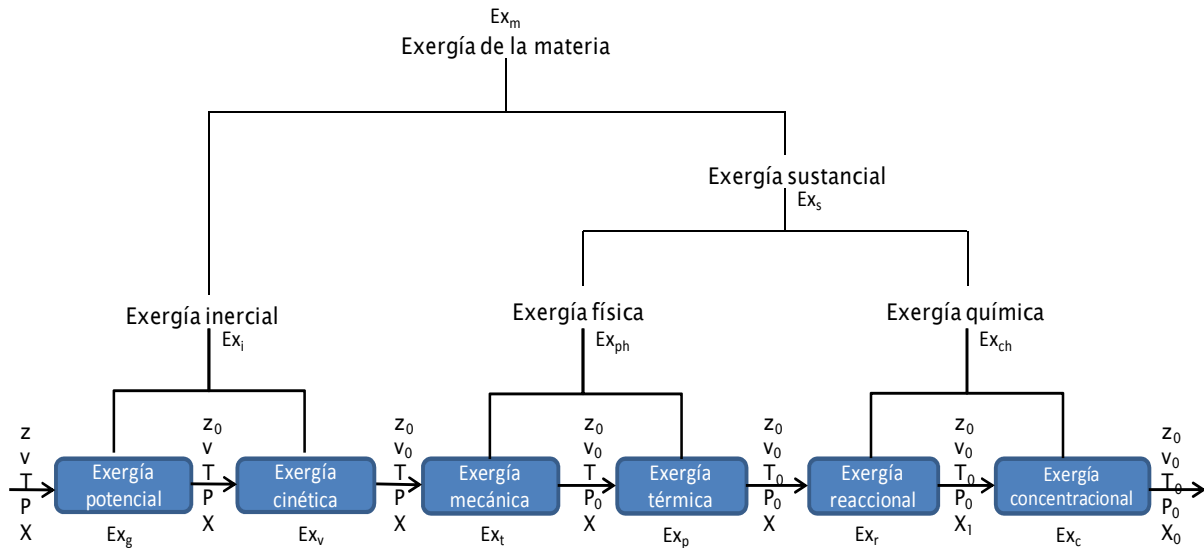
Figura 2.3. Exergía sustancial. Fuente: Rivero, 2010
