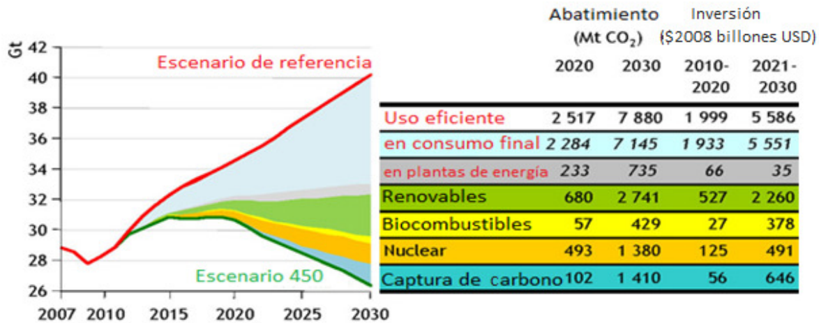
Figura 1.6. Abatimiento de emisiones de CO 2 . Fuente: IEA, 2008
