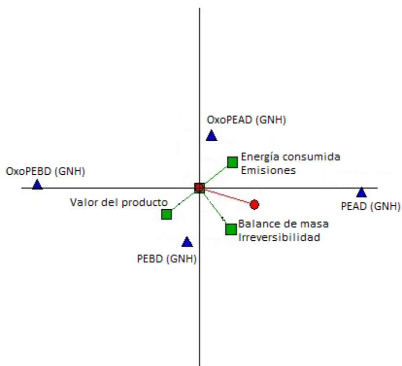
Figura 5.7. Plano GAIA para las opciones provenientes del gas natural húmedo
