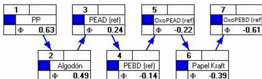
Figura 5.4. Orden jerárquico (“ranking”) completo, sin aquellas opciones provenientes del gas natural húmedo. (PEBD (ref)= polietileno de baja densidad proveniente de petróleo crudo, PEAD (ref)= polietileno de alta densidad proveniente de petróleo crudo, PP= polipropileno, Oxo-PEBD (ref)= polietileno
