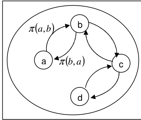
Figura 4.7. Gráfico de índices de preferencias agregadas. Fuente: Brans y Mareschal, 2002
