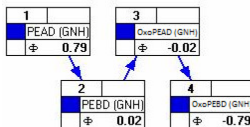
Figura 5.6. Orden jerárquico ("ranking") completo para las opciones provenientes del gas natural húmedo. (PEBD (GNH)= polietileno de baja densidad proveniente de gas natural húmedo, PEAD (GNH)= polietileno de alta densidad proveniente de gas natural húmedo, Oxo-PEBD (GNH)= polietileno de baja
