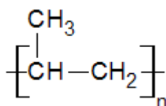
Figura A1.6. Estructura repetitiva del polipropileno
