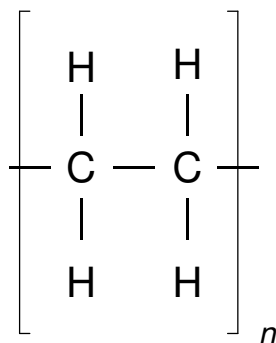
Figura A1.1. Unidad repetitiva del polietileno
