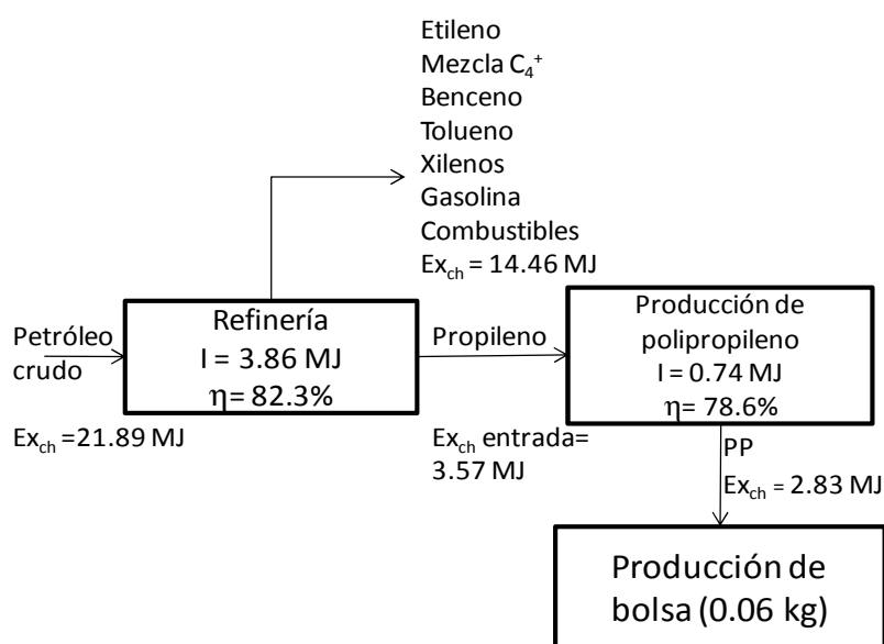
Figura 5.10. Diagrama de exergía para el ciclo de vida de una bolsa de polipropileno
