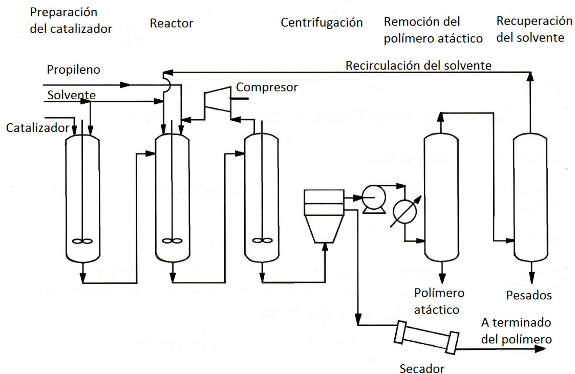
Figura A1.8. Polipropileno por polimerización en suspensión. Fuente: Wells, 1991
