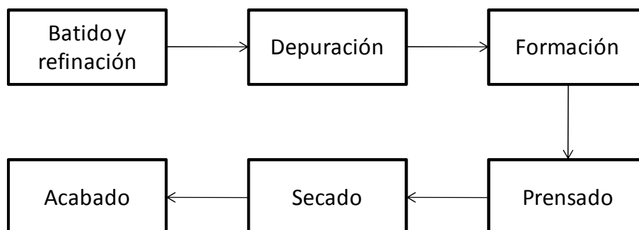
Figura A1.12. Representación de las principales operaciones que se realizan en la elaboración de papel Kraft. Fuente: Jiménez, 2005
