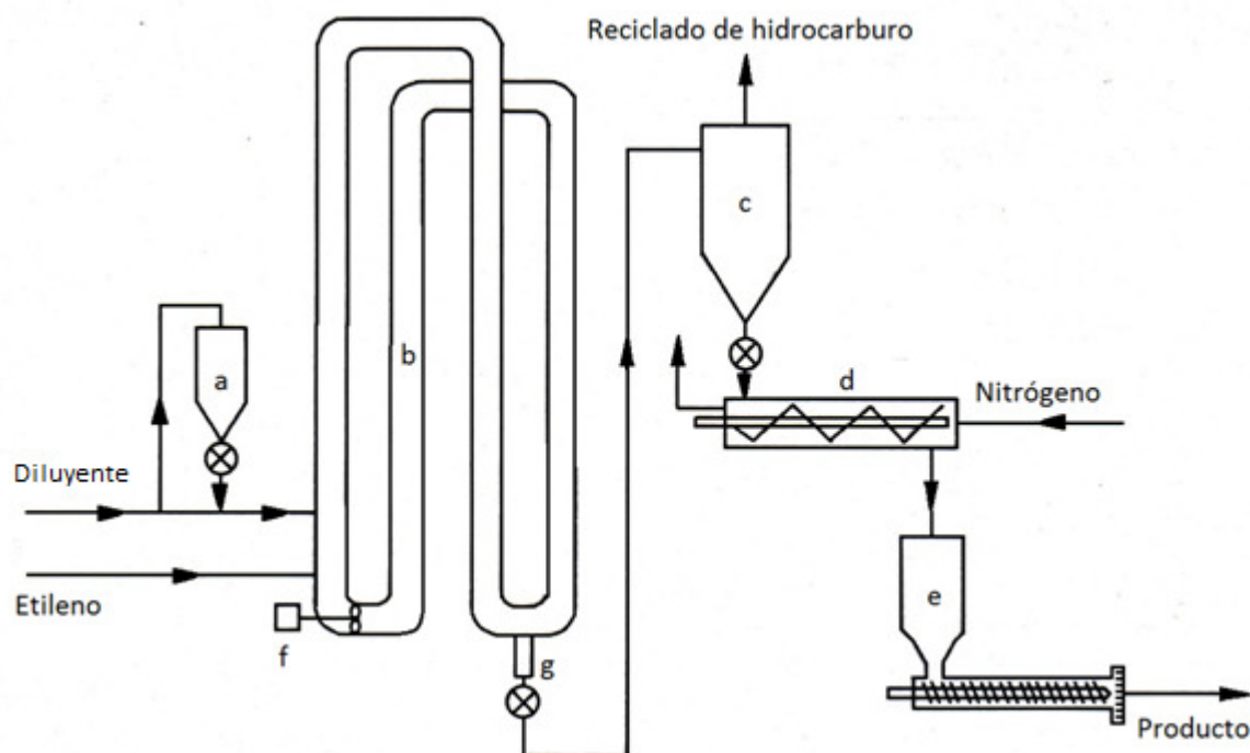
Figura A1.2. Proceso de partícula de Phillips. a) Tolva de catalizador y válvula de alimentación; b) reactor de doble lazo; c) tanque “flash”; d) secador de purga; e) extrusor; f) impulsor; g) sedimentador. Fuente: Ullmann, 1989
