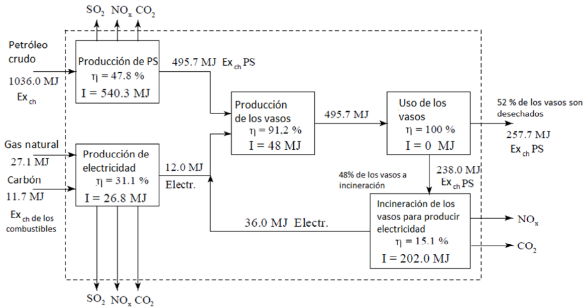
Figura 3.2. Diagrama de exergía para el ciclo de vida de 3000 vasos de poliestireno. Fuente: Cornelissen, 1997
