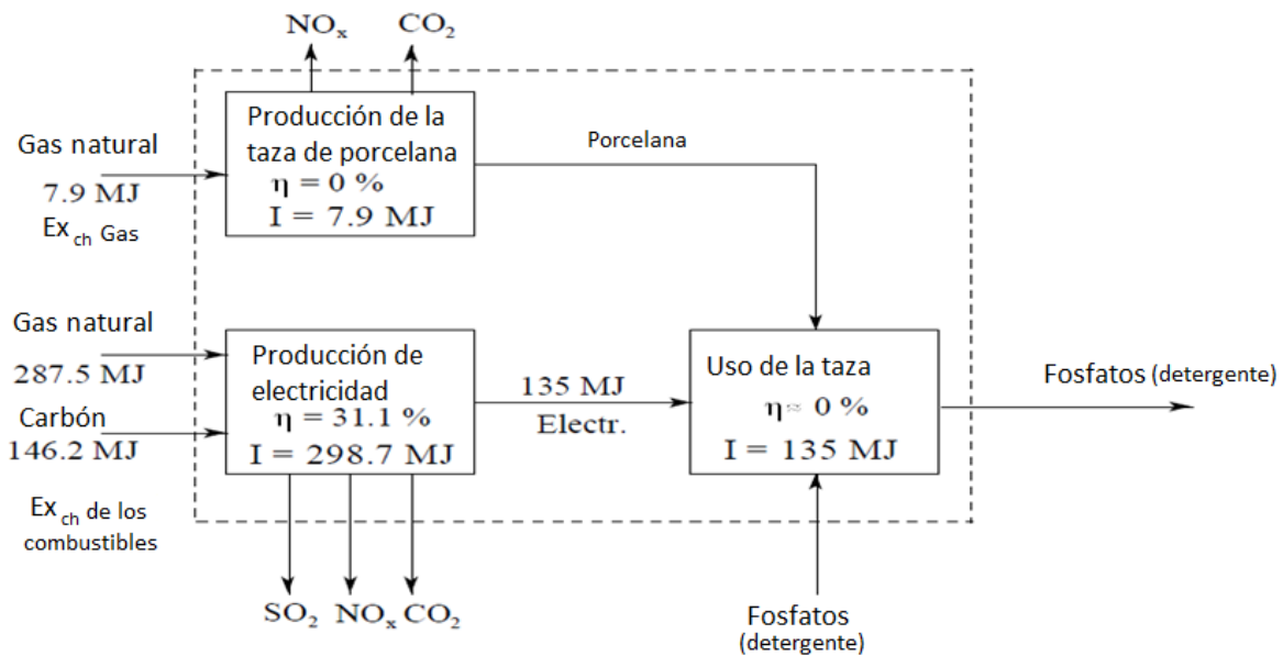
Figura 3.3. Diagrama de exergía para el ciclo de vida de una taza de porcelana. Fuente: Cornelissen, 1997
