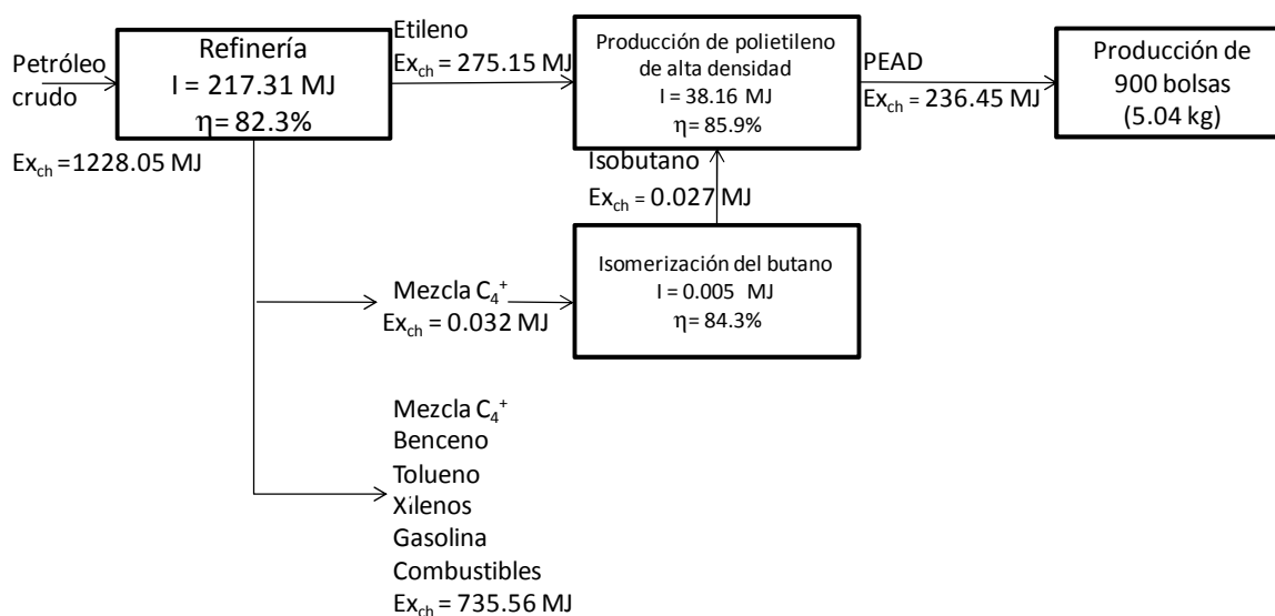
Figura 5.12. Diagrama de exergía para el ciclo de vida de 900 bolsas de polietileno de alta densidad a partir de petróleo crudo
