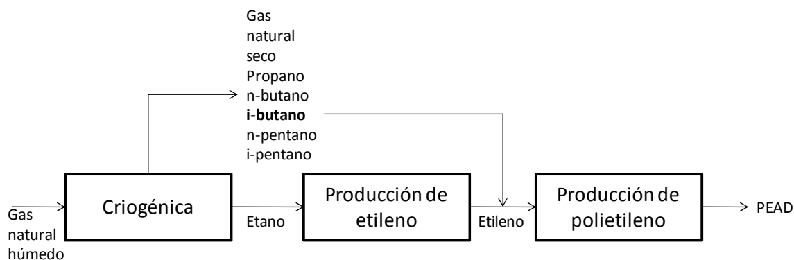
Figura A2.2. Cadena de producción de polietileno de alta densidad a partir de GNH (el eteno es conocido coloquialmente como etileno)
