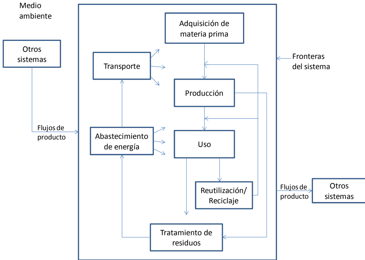
Figura 3.1. Ejemplo de un sistema de producto para un ACV. Fuente: ISO 14040:2006
