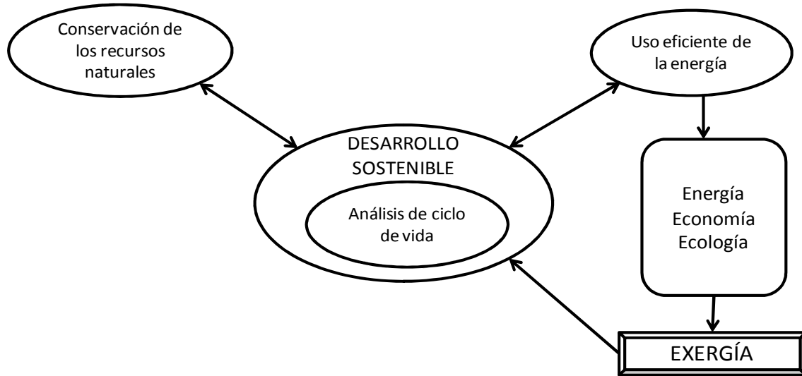
Figura 4.1. Marco de referencia. Fuente: Elaboración propia
