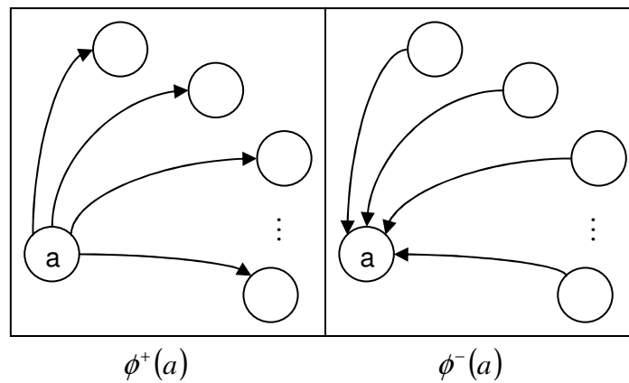
Figura 4.8. Flujos de categorías de PROMETHEE. Fuente: Brans y Mareschal, 2002
