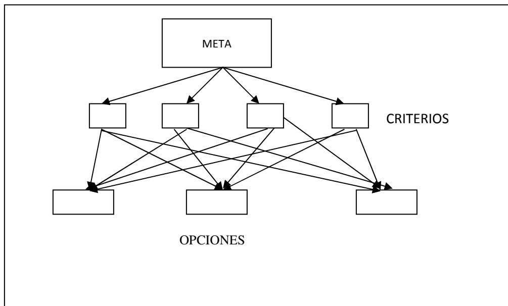
Figura 4.5. Jerarquía de tres niveles. Fuente: Escobar-T., 2009
