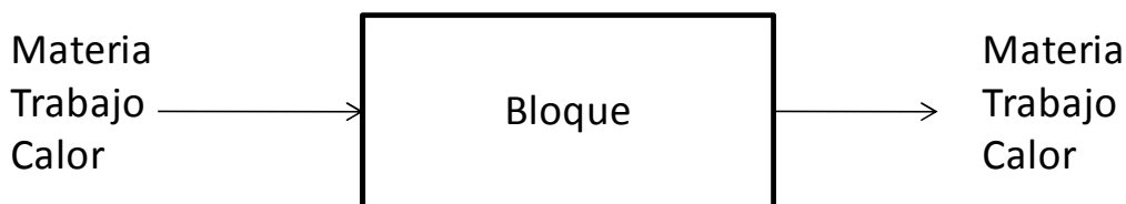
Figura 4.3 Entradas y salidas de un bloque. Fuente: Rivero, 1994.
