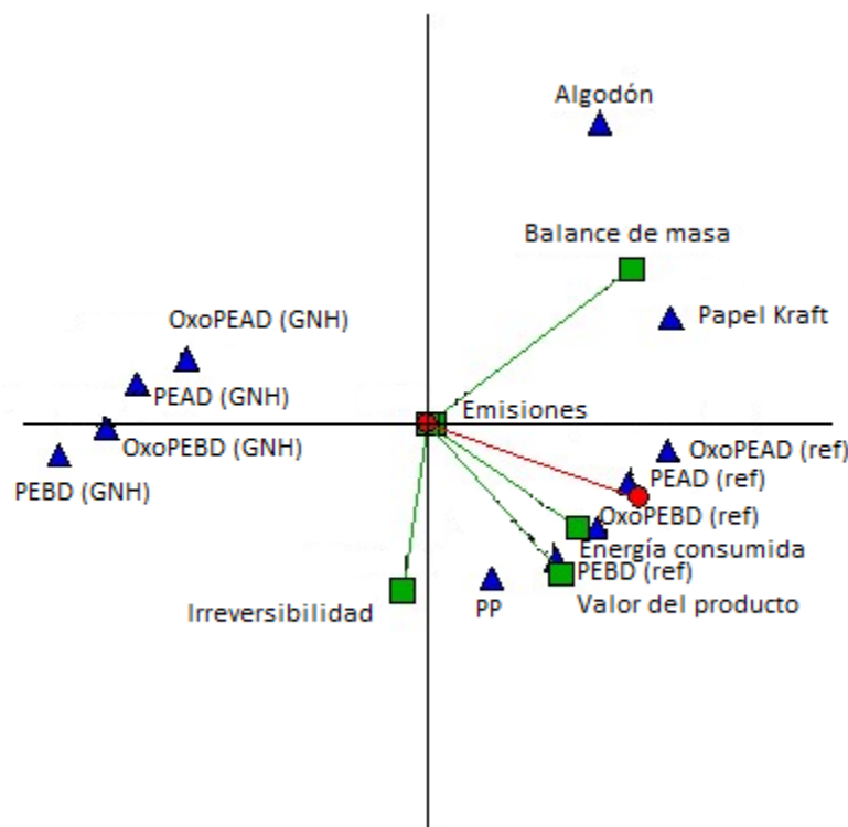
Figura 5.9. Plano GAIA, en relación con las toneladas de material
