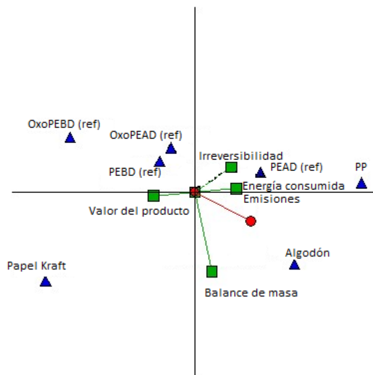
Figura 5.5. Plano GAIA para las opciones, excluyendo aquellas provenientes del gas natural húmedo
