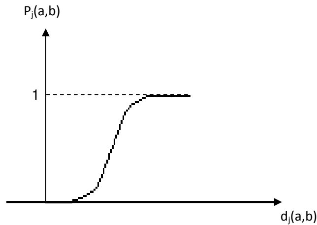
Figura 4.6. Función de preferencia. Fuente: Brans y Mareschal, 2002
