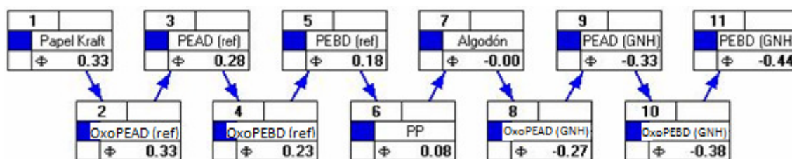
Figura 5.8. Orden jerárquico ("ranking") completo, en relación con las toneladas de material. (PEBD (GNH)= polietileno de baja densidad proveniente de gas natural húmedo, PEBD (ref)= polietileno de baja densidad proveniente de petróleo crudo, PEAD (GNH)= polietileno de alta densidad proveniente de gas natural húmedo, PEAD (ref)= polietileno de alta densidad proveniente de petróleo crudo, PP= polipropileno, Oxo-PEBD (GNH)= polietileno de baja densidad (con agente degradante) proveniente de gas natural húmedo, Oxo-PEBD (ref)= polietileno de baja densidad (con agente degradante) proveniente de petróleo crudo, Oxo-PEAD (GNH)= polietileno de alta densidad (con agente degradante) proveniente de gas natural húmedo, Oxo-PEAD (ref)= polietileno de alta densidad (con agente degradante) proveniente de petróleo crudo)
