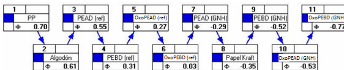
Figura 5.2. Orden jerárquico (“ranking”) completo para las opciones propuestas. (PEBD (GNH)= polietileno de baja densidad proveniente de gas natural húmedo, PEBD (ref)= polietileno de baja densidad proveniente de petróleo crudo, PEAD (GNH)= polietileno de alta densidad proveniente de gas natural húmedo, PEAD (ref)= polietileno de alta densidad proveniente de petróleo crudo, PP= polipropileno, Oxo-PEBD (GNH)= polietileno de baja densidad (con agente degradante) proveniente de gas natural húmedo, Oxo-PEBD (ref)= polietileno de baja densidad (con agente degradante) proveniente de petróleo crudo, Oxo-PEAD (GNH)= polietileno de alta densidad (con agente degradante) proveniente de gas natural húmedo, Oxo-PEAD (ref)= polietileno de alta densidad (con agente degradante) proveniente de petróleo crudo)
