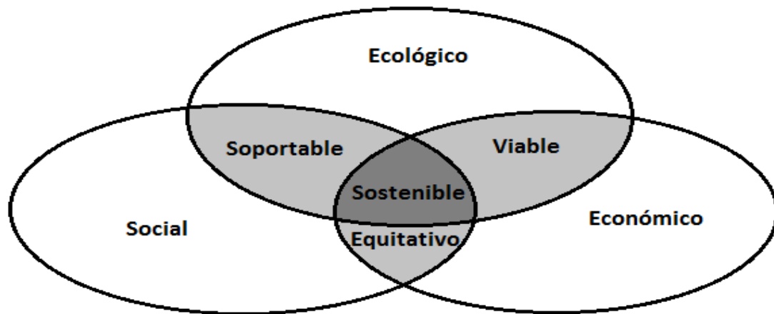
Figura 1.1. Elementos principales para el desarrollo sostenible. Fuente: Página electrónica de la FAO
