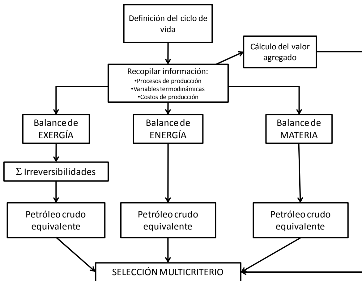
Figura 4.2. Metodología propuesta para evaluar materiales con la misma función. Fuente:
