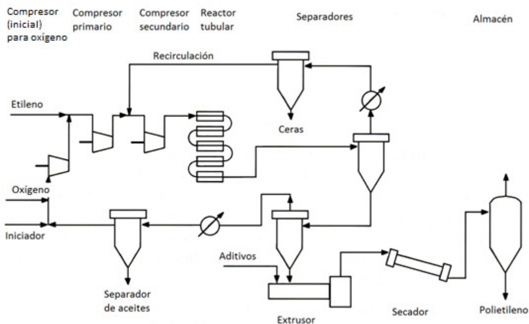
Figura A1.3. Obtención de polietileno de baja densidad por medio de la polimerización de etileno en un reactor tubular. Fuente: Wells, 1991
